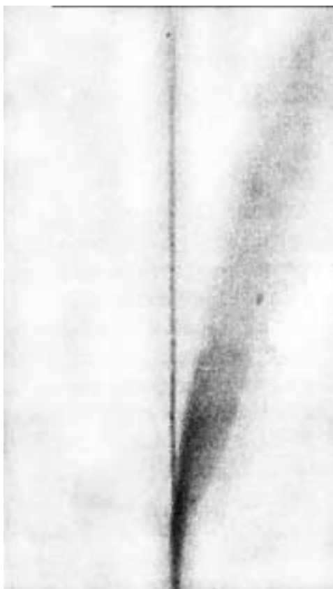
6. ábra. Mágneses mezőben eltérített \beta - és \gamma -sugárzás „fénycépe”
